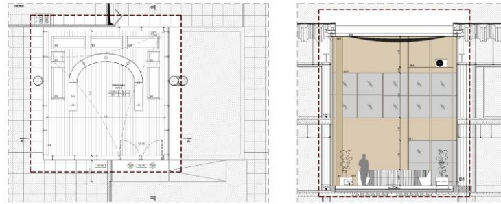
PLANTA DO PISO 0 ESCALA 1:100
