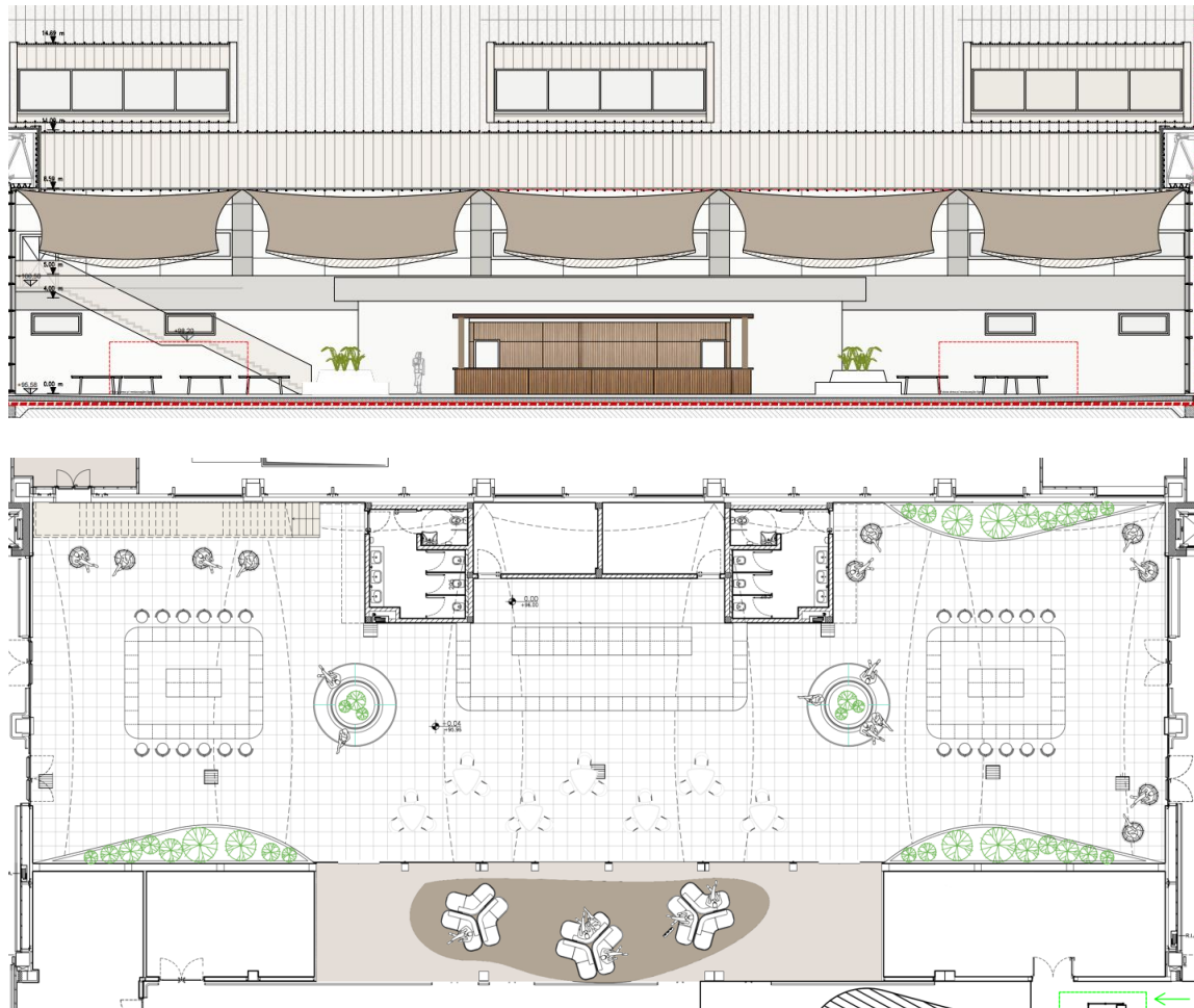
QW-RAI 1A – NOVO PÁTIO COM OFERTA COMERCIAL
